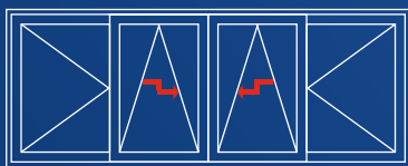
4-teiliges Element mit 2 Schiebeflügeln und 2 Drehflügeln
